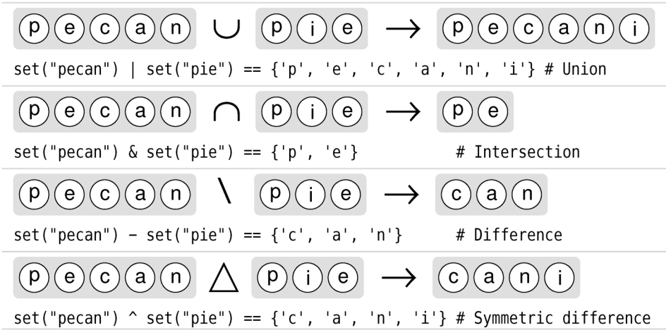
图 3-4 标准的集合操作符
