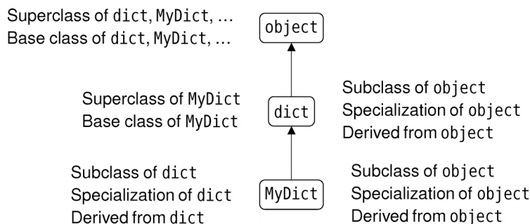
图 6-1 一些面向对象术语
