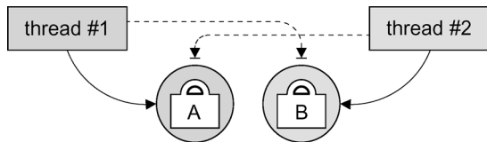
图 10-2 死锁：两个或更多阻塞的线程尝试请求彼此的锁
