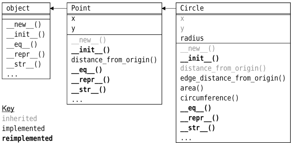
图 6-3 Circle 类的继承体系
