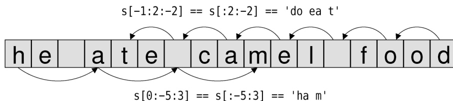
图 2-4 序列分片与步距
