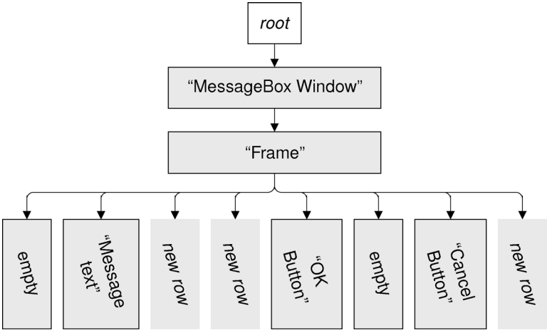
图 14-14 分析后 messagebox.blk 文件的块及其孩子
