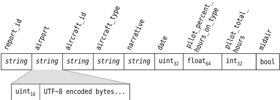
图 7-3 二进制航空器事故记录格式
