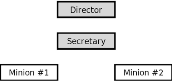
图 14-9 hierarchy.svg 文件
