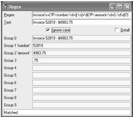
图 15-8 regex 程序
