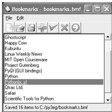
图 15-4 Bookmarks 程序
