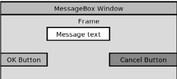
图 14-11 messagebox.svg 文件
