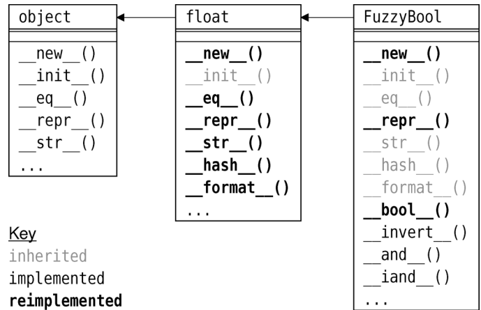
图 6-5 替代的 FuzzyBool 类的继承体系
