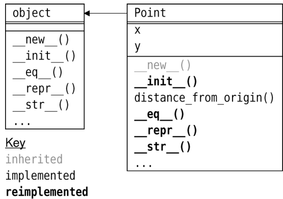
图 6-2 Point 类的继承体系
