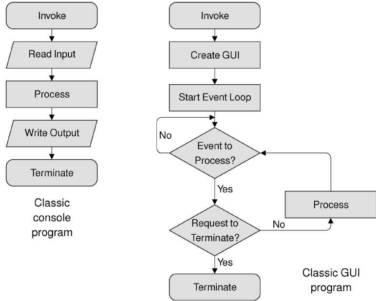
图 15-1 控制台程序对比 GUI 程序
