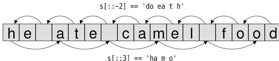
图 2-3 序列步距
