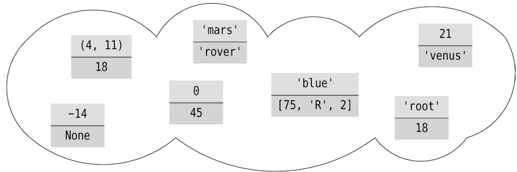
图 3-5 字典
