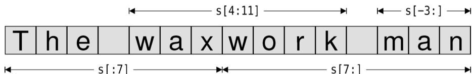
图 2-2 序列分片
